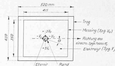
Abb. 2. Anordnung zum Lochversuch. Gesteuerte Punkte 36, d. h. alle 10°. Gesetz der Randspannungsverteilung:
