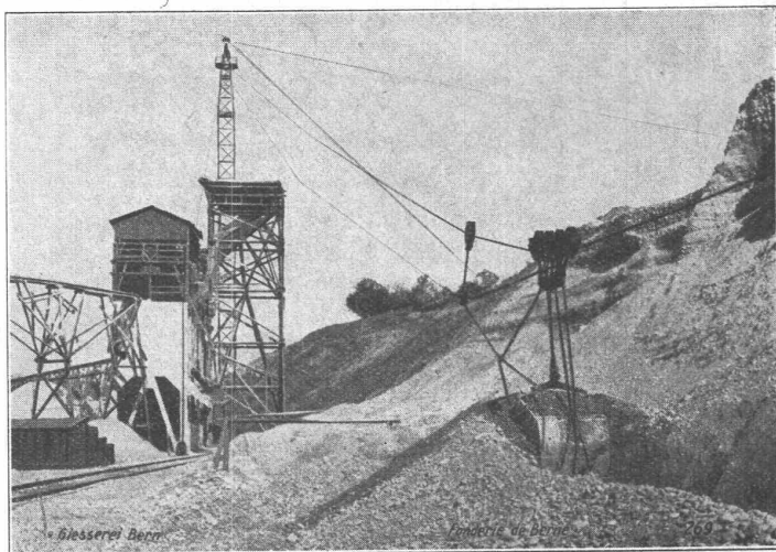
Kabelbaggeranlage Olten.
