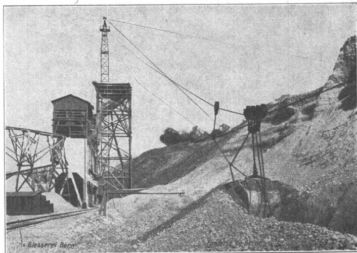
Kabelbaggeranlage Olten.
