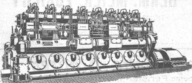
300 PS Schiffsdieselmotor mit Öl-Druck-Wendegeriebe
