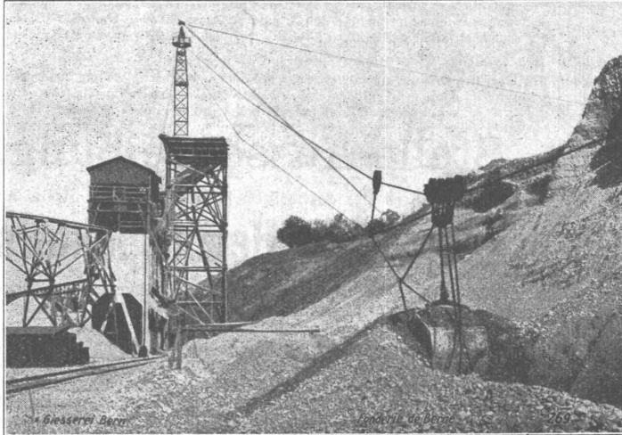
Kabelbaggeranlage Olten.
