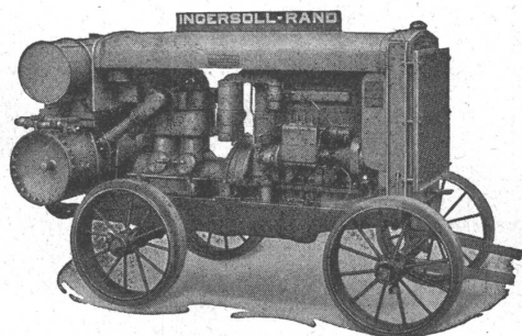
Rohölkompressor 20/26 PS.
