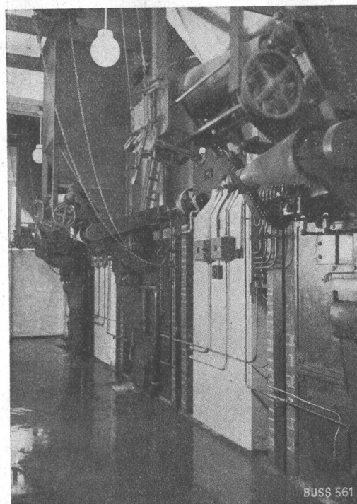
Drei Spezial-Heisswasserkessel mit mechanischer Beschickung, System Groll, + Patent, Fabrikat Buss A. G.
