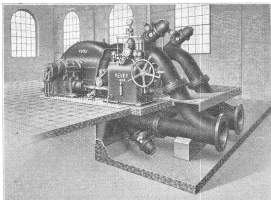
Doppel Pelton-Turbine des Kraftwerkes Sernf-Niederembach. Gefälle 215 m, Tourenzahl 500 p. min., 3400 PS.
