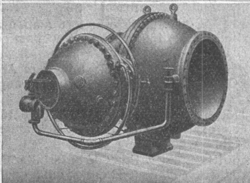
Oben: Keilschieber 2500 mm Nennweite, 7 at Druck, für ein Kraftwerk in Spanien. — Unten: Drehschieber 1600 mm Nennweite, 15 at Druck, für ein automatisches Kraftwerk in Deutschland.
