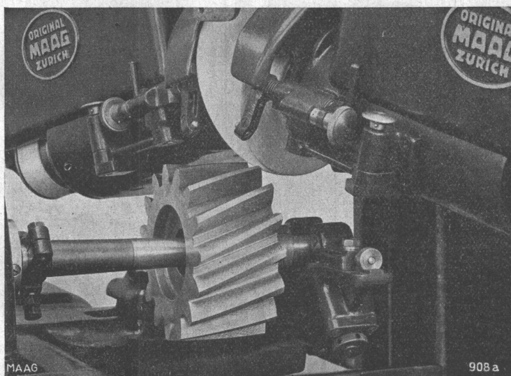
MAAG-ZAHNRADSCHLEIFMASCHINE für Stirn- und Schraubenverzahnungen Schleifgenauigkeit bis 0,002 mm.
