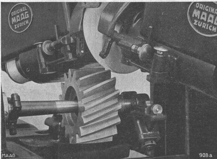
MAAG-ZAHNRADSCHLEIFMASCHINE für Stirn- und Schraubverzahnungen Schleifgenauigkeit bis 0,002 mm.
