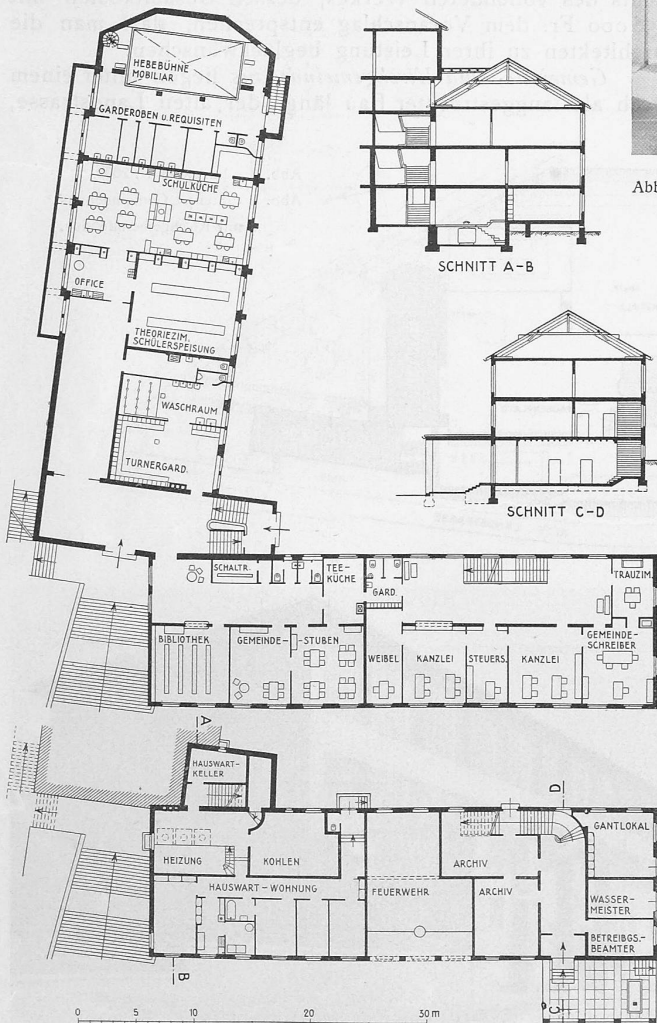
Abb. 5 und 6. Grundrisse und Schnitte. — Masstab 1 : 600.
