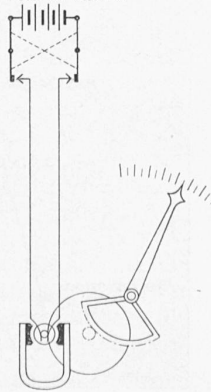
Abb. 2. Schema des Fernmelders.
