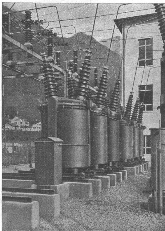
150 kV Oelschaltergruppen
