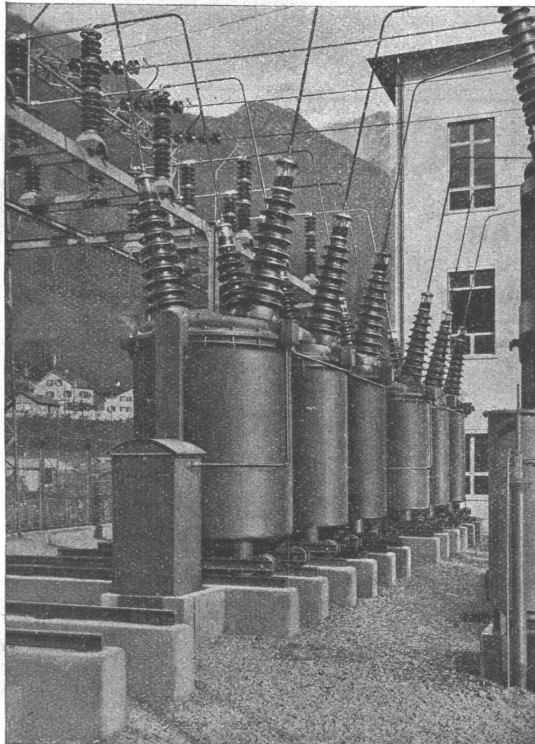
150 kV Oelschaltergruppen
