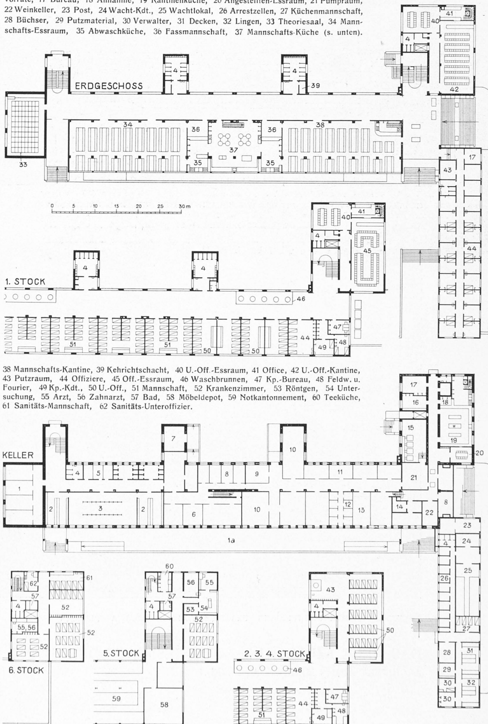
Abb. 3. Südostansicht — Abb. 4 bis 9. Grundrisse 1:800 der neuen Infanterie-Kaserne.
