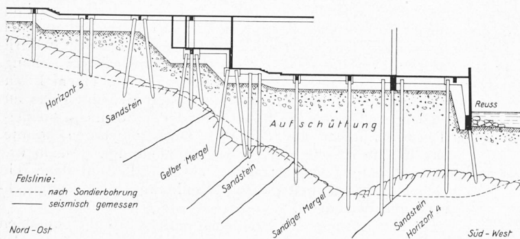
Abb. 1. Profil in der Längsaxe der Kirche, senkrecht zur Reuss. — Masstab 1 : 500.
