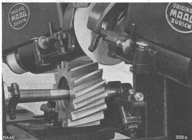
Maag-Schraubenrad-Schleifmaschine
