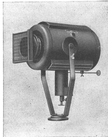
Vorbühnen-Scheinwerfer
