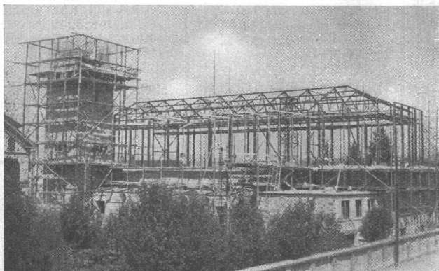
Kirchenbau Niederuzwil
