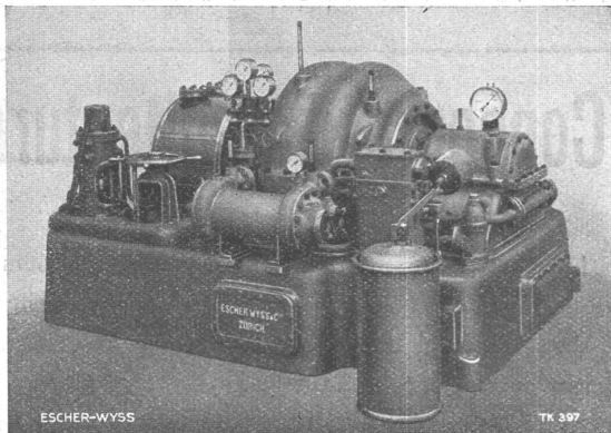
Koks-Gasgebläse mit Dampfturbinenantrieb
