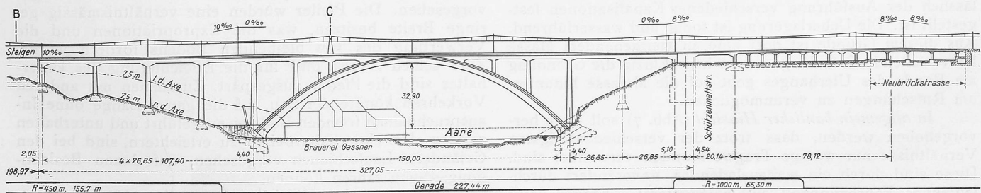
Abb. 4. Projektierter Aareübergang und Schützenmattviadukt der S. B. B. mit Strassenunterführungen. — Masstab 1 : 2500.
