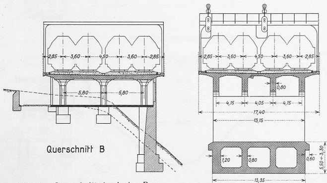
Abb. 3. Querschnitt durch den Bau an der Lorrainehalde. — 1 : 500.
