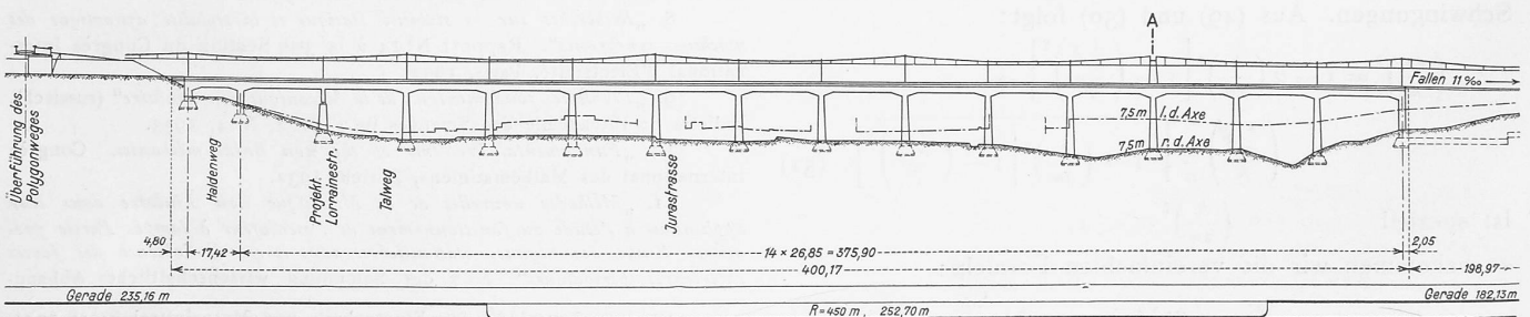
Abb. 1. Projektierter Viadukt über die Talwegmulde, Masstab 1 : 2500, mit Terrainlinien je 7,5 m rechts und links der Axe.
