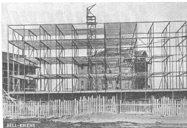
Stahlskelett des Pavillon Suisse in der Cité Universitaire, Paris
