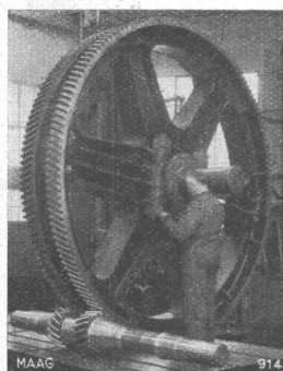
Maag-Pfeilradgetriebe für Förderanlage, Charbonnages Elisabeth, Auvélaix Belgien. (Ritzelverzahnung, gehärtet und geschliffen.)
