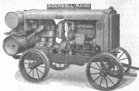
Rohölkompresseur 20/26 PS.
