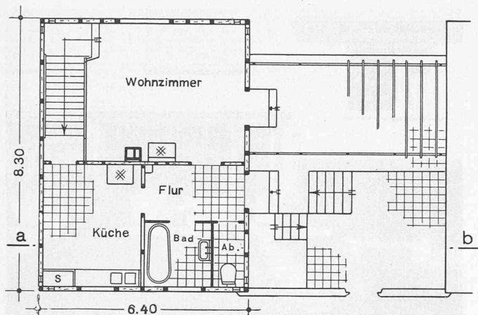
Abb. 10. Haus 2, Prof. Paul Schmittner. — Erdgeschoss 1 : 150 (oben SO-Front).
