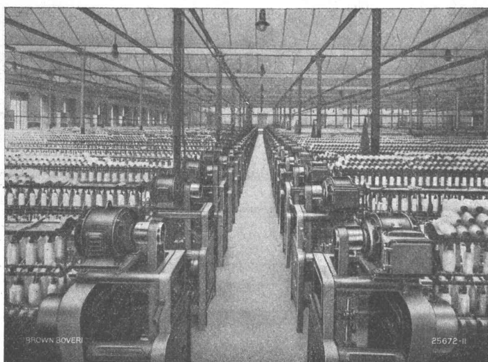
Einzelantrieb v. Ringspinnmaschinen durch aufgebauete Kurzschlussankermotoren.
