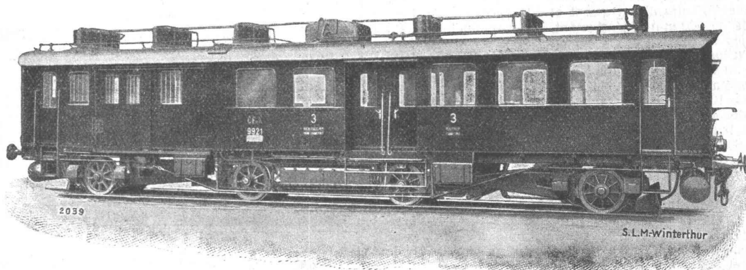
300 PS Dieseltriebwagen im Betrieb auf der Strecke Glarus-Uznach der S. B. B., ausgerüstet mit Geschwindigkeitswechselgetrieben System „S. L. M.-Winterthur“.
