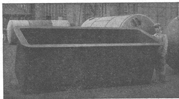
VERZINKUNGSKESSEL für unsere Abt. Verzinkerei vor dem Versand i Vm Werk
