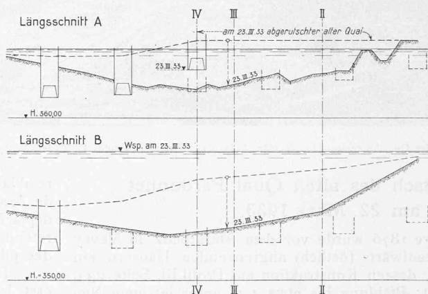
Abb. 6. Längsschnitte in der innern und äussern Pfeileraxe. — Masstab 1 : 800.
