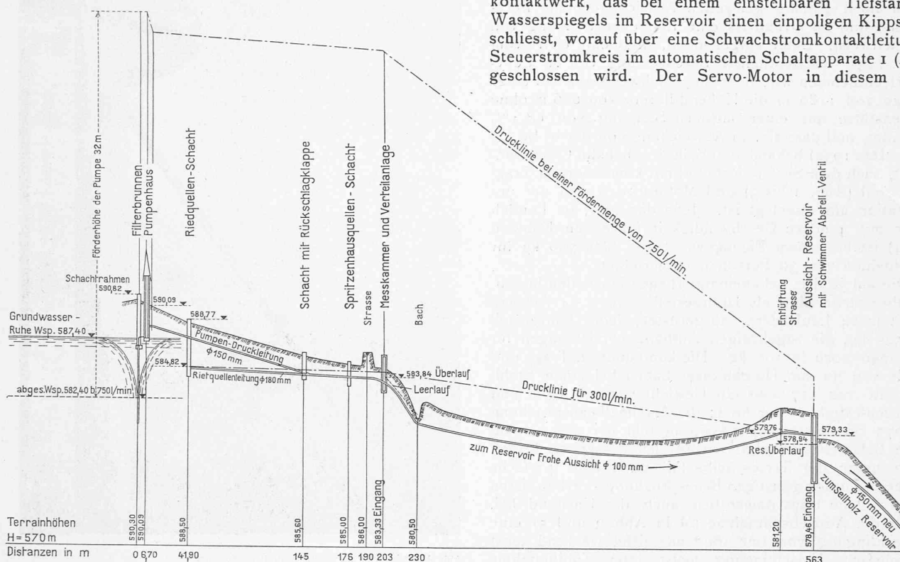
Abb. 1. Längenprofil der Grundwasser-Ergänzungsanlage der Wasserversorgung Herrliberg-Erlenbach. — Masstab für die Längen 1 : 4000, für die Höhen 1 : 400.
