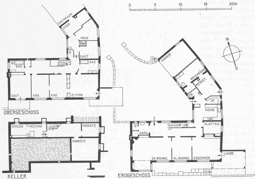
Abb. 6. Grundrisse des Wohnhauses „zum Höfli“; 1 : 400. — Arch. Moser & Kopp, Zürich.
