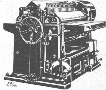
Hochleistungs-Dickenhobelmaschine Typ DH
