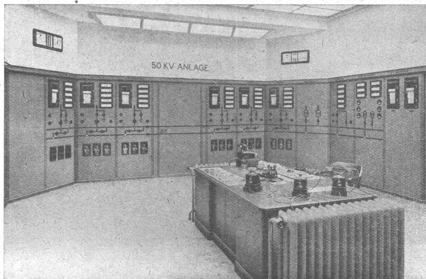
Kommandosaal im Unterwerk Grynau der N. O. K., Baden.
