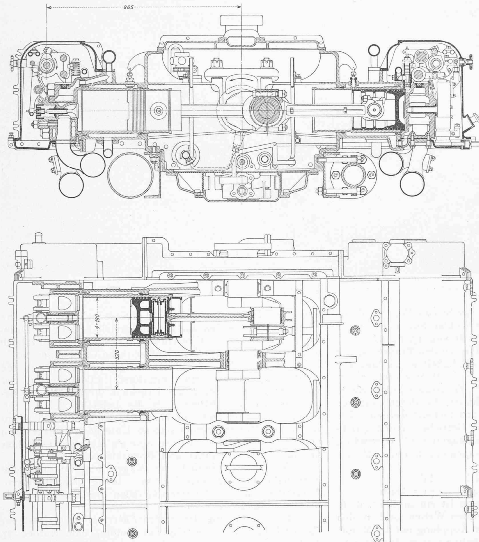
Abb. 3. Horizontaler Zwölfzylinder-Dieselmotor von 300 PS des Triebwagens System „S. L. M. Winterthur.“
