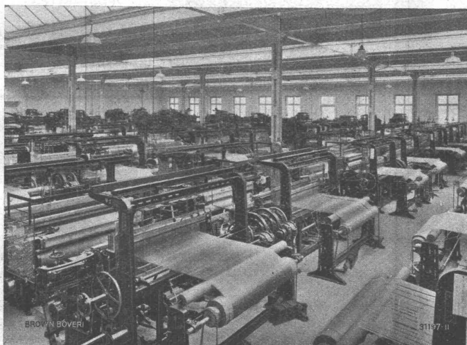
Brown Boveri-Rüti Zahnradantrieb für Seidenstühle.
