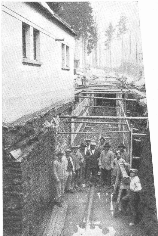
Unterirdische Transport- und Fernheizungskanäle Kantonsspital - Neubau Luzern. • Bauleitung: Bureau des Kantonsbaumeisters für Spitalbauten. • Unternehmer: J. Pfisterer & Galli Söhne, Luzern.
