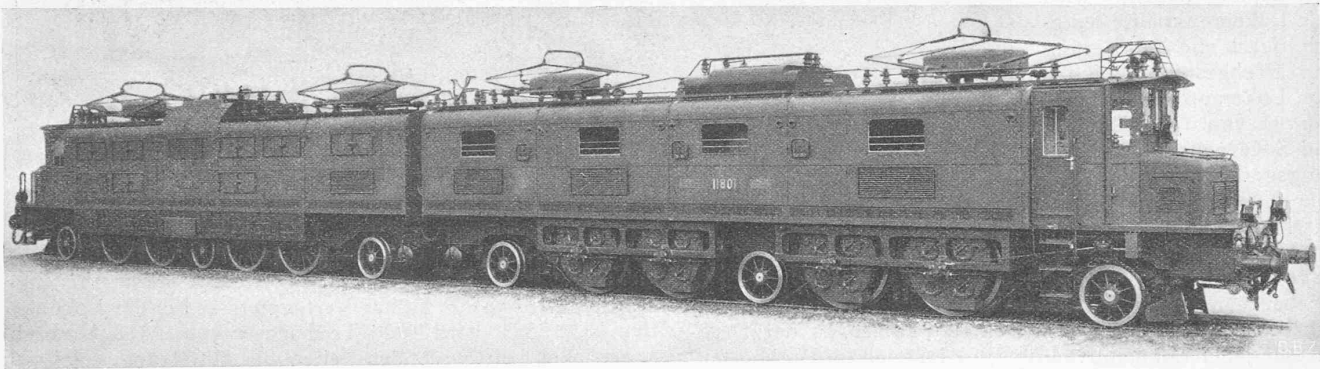
Abb. 1. Ae 8/14 Lokomotive Nr. 11801 für die Gotthardlinie. Ausführung mit BBC-Antrieb. Dienstgew. 244,0 t, Adhäsionsgew. 156,2 t. Dauerleistung 7000 PS bei 61 km/h.
