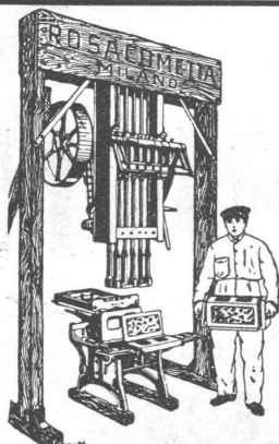
Leichteste Hohlsteine für Decken in Eisenbeton
