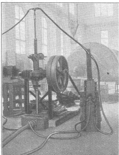
Konsolidation eines Generatorenfundamentes mit Hilfe von Kernbohrungen. Verankerungsseilen und Injektionen.
