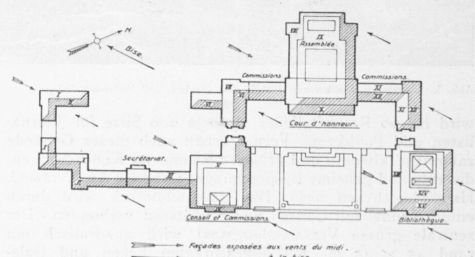
Abb. 13. Gegenvorschlag der Gruppe Gebr. Sulzer. — 1:4500.
