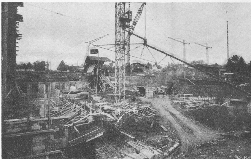
Abb. 8. Bâtiment du Conseil. Foundation. Giessturm 67 m hoch. (30. Oktober 1931.) Links der Anschluss an den Sekretariatsflügel, im Hintergrund Krane von Abb. 3.
