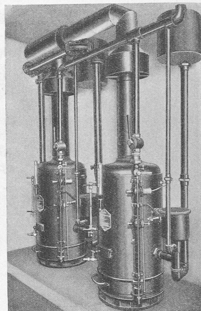
Abb. 8 und 9. Kupferner Gasheizkessel der Askaniewerke Berlin.
