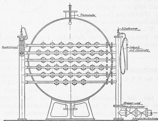
Abb. 7. Längsschnitt und Vorderansicht des Hochdruck-Gaskessels der Gebr. Körting in Körtingsdorf.
