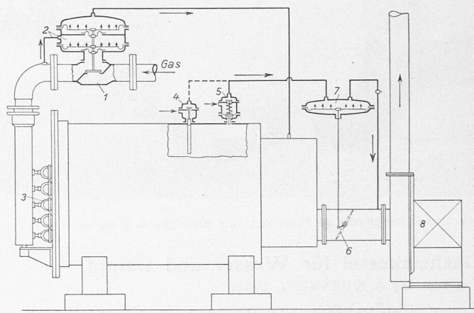
Abb. 3. Generelles Regulierschema zum Bamag-Gaskessel. — 1 Gasreguliertventil, 2 Gasdruckregler, 3 Brenner, 4 Temperatur-Steuerventil, 5 Druck-Steuerventil, 6 Drosselklappe, 7 Steuermembran für Zug, 8 Abgasventilatoren.
