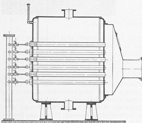
Abb. 7. Längsschnitt und Vorderansicht des Hochdruck-Gaskessels der Gebr. Körting in Körtingsdorf.
