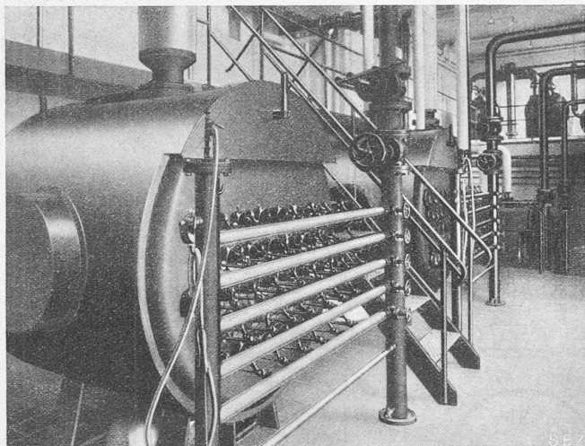
Abb. 6. Ausgeführte Anlage mit Körting-Gaskessel.
