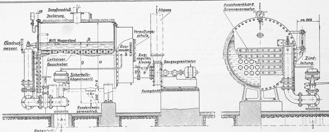
Abb. 2. Längs- und Querschnitt durch einen Gas-Hochdruckdampfkessel der Bamag-Méguin A.-G., Berlin.
