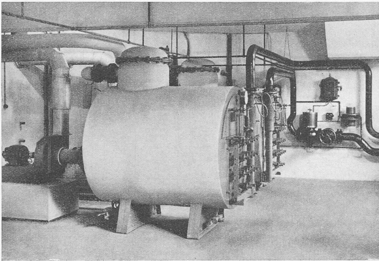
Abb. 1. Gas-Dampfkessel der Firma Rud. Otto Meyer (ROM) in Sambury.
