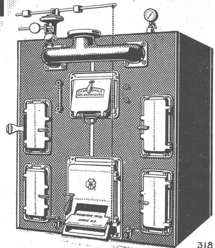
"IDEAL" GLIEDERKESSEL SÉRIE MF
