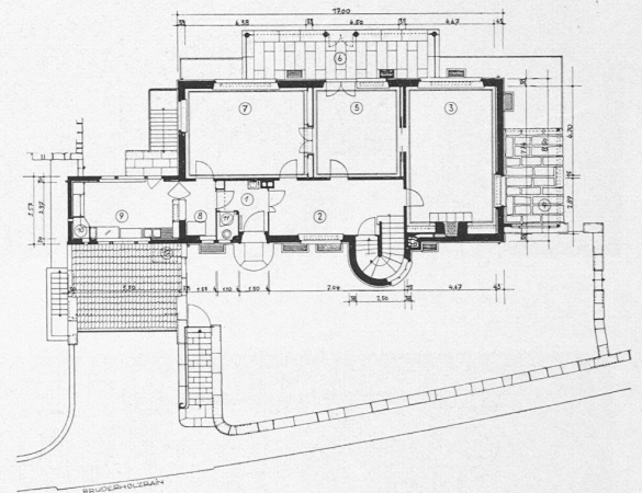
Abb. 6. Erdgeschoss. — 3 Wohnzimmer, 5 Salon, 7 Esszimmer, 9 Küche.
