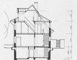
Abb. 9 bis 11. Grundrisse und Schnitt, 1 : 400.
