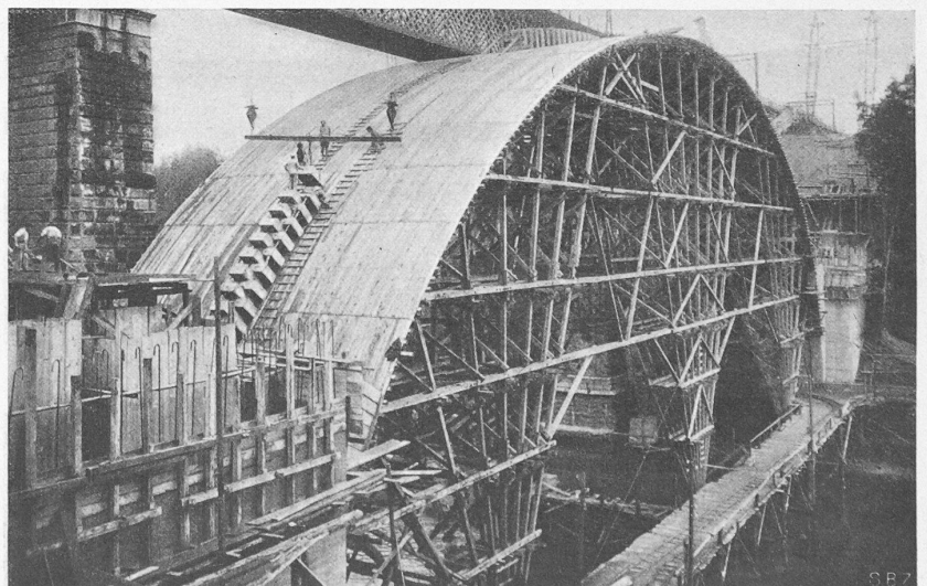
Abb. 23. Beginn der Gewölbemauerung, erstes Element. (3. November 1928.)
