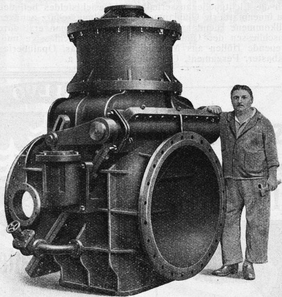
RÜCKSCHLAG-VENTIL, 1000 mm Lichtweite
