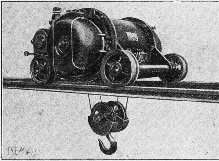
Zweischienenkatze für Laufkran.
