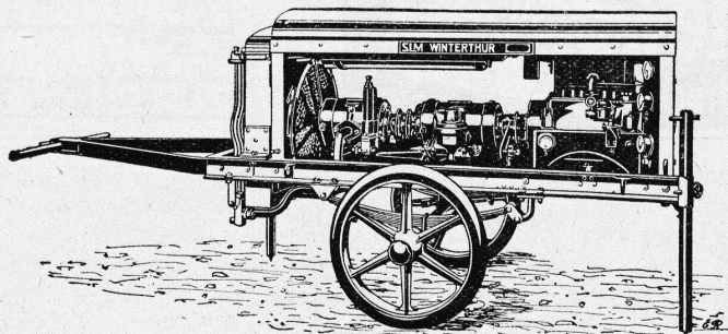
Fahrbare Kompressoranlage „S. L. M. Winterthur“ für Drücke bis 7 Atm.
