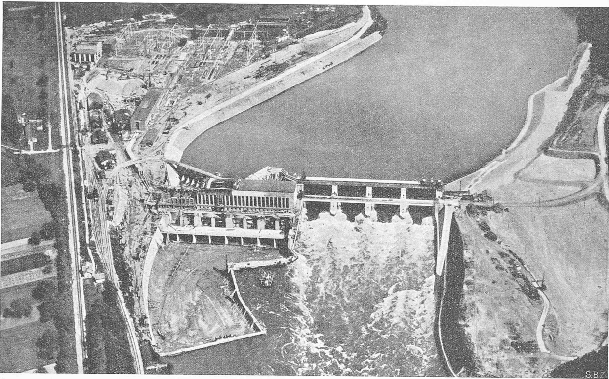
Abb. 5. Fliederbild aus Westen auf die Gesamtanlage des Kraftwerkes Ryburg-Schwörstadt im Bauzustand Ende Mai 1930.
