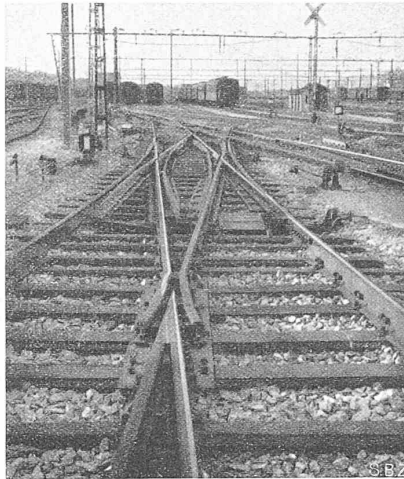
Abb. 19. Normale Kreuzungsweiche 1 : 8.
