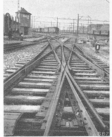
Abb. 20. Steile Kreuzungsweiche 1 : 6,5.
