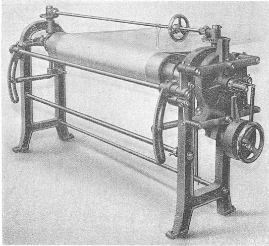
Abb. 14. Kettbaumgestell mit selbsttätiger Ablassvorrichtung.
