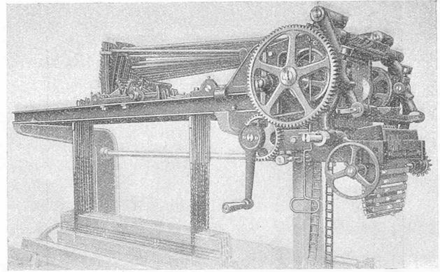
Abb. 17. Tiefliegende Doppelhub-Schaffmaschine mit Hubexzentrern.
