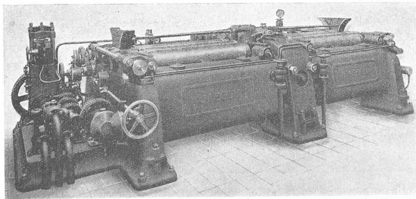
Abb. 9. Stranggarn-Mercerisiermaschine von vorne, in Arbeitstellung.
