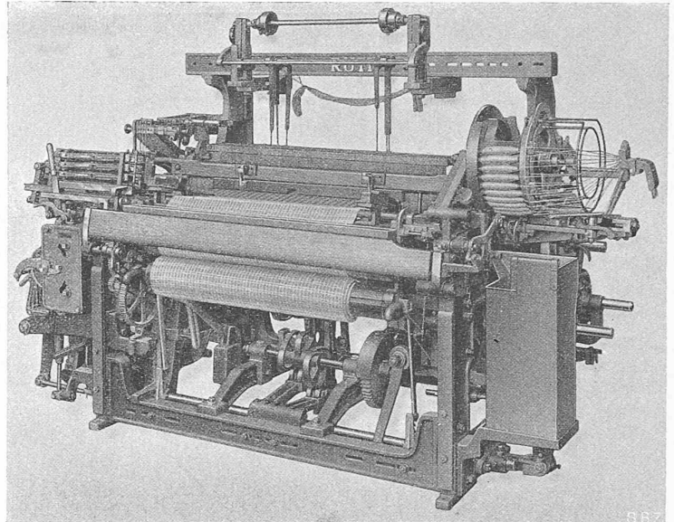
Abb. 15. Vierschütziger Baumwoll-Automat, mit unterteilter Northrop-Trommel. M.-F. Rütli.
