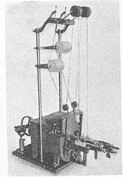
Abb. 7. Einzelkopf der Kreuz-Spulmaschine für Schuss-Spulen mit konischen Enden.
