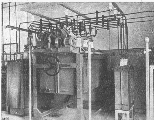
Installation de réglage automatique d'un feeder triphasé de 1500 kVA, 8400 \pm 10 % Volts, 50 pér/sec.
