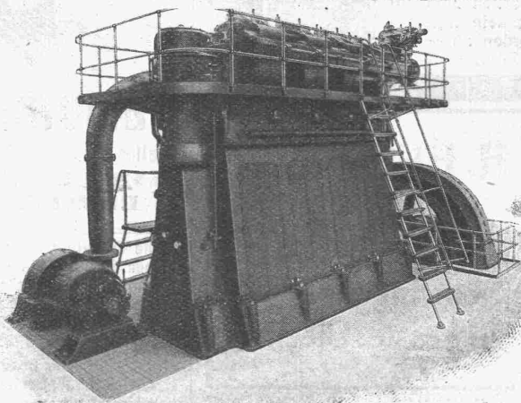
1150 PSe „S. L. M.-Winterthur“-Dieselmotor mit Büchi-Abgas- turbinaufladung
