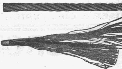
„Tru-Lay“-Drahtseil nicht abgebunden.
