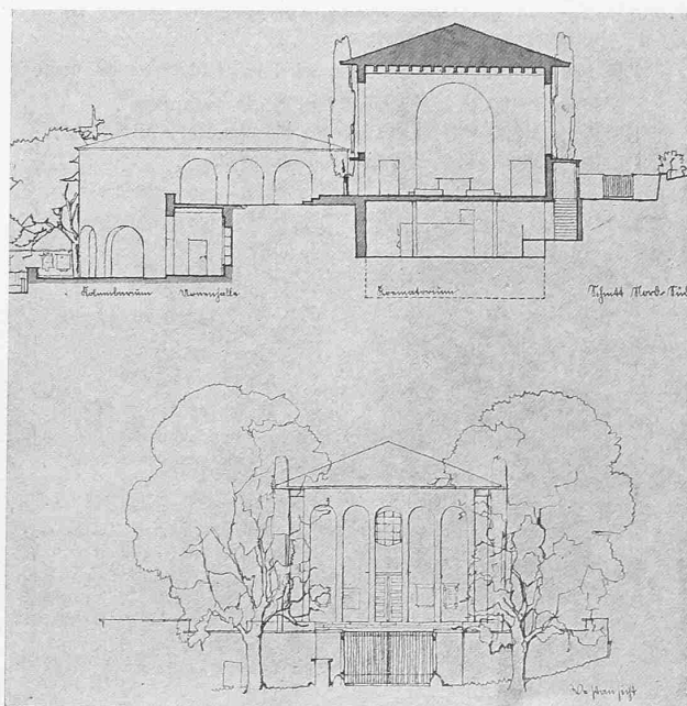
Querschnitt und Ansicht des Krematoriums. — 1 : 400.
