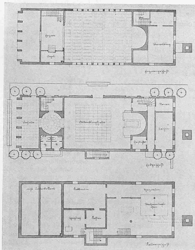
I. Preis, Entwurf Nr. 2, — Grundrisse des Krematoriums. — 1 : 400.
