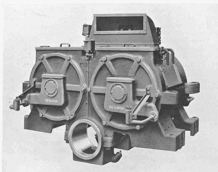
Abb. 4. Doppelmotor von 2 x 450 PS Einstundenleistung.
