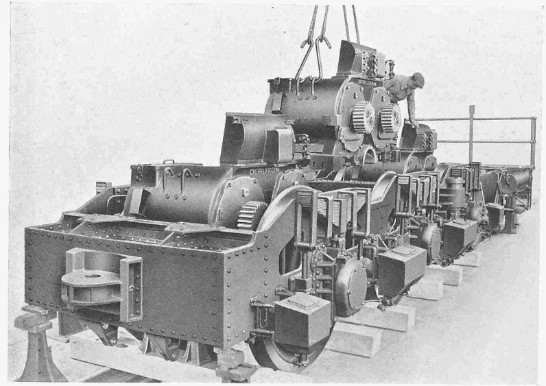
SCHNELLZUGSLOKOMOTIVE VON 5400 PS DER P. L. M.
