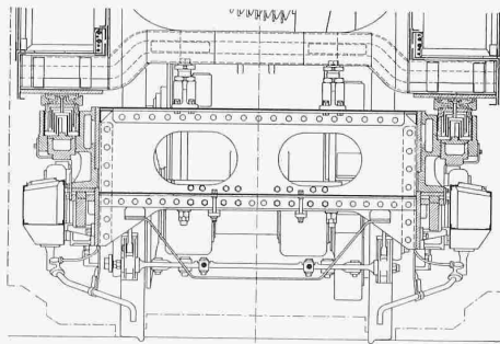
SCHNELLZUGSLOKOMOTIVE VON 5400 PS DER P. L. M.
