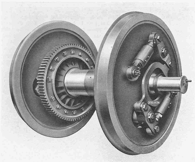
Abb. 2. Triebbradsatz mit Zahnrad, Hohlwelle und Federkupplung.
