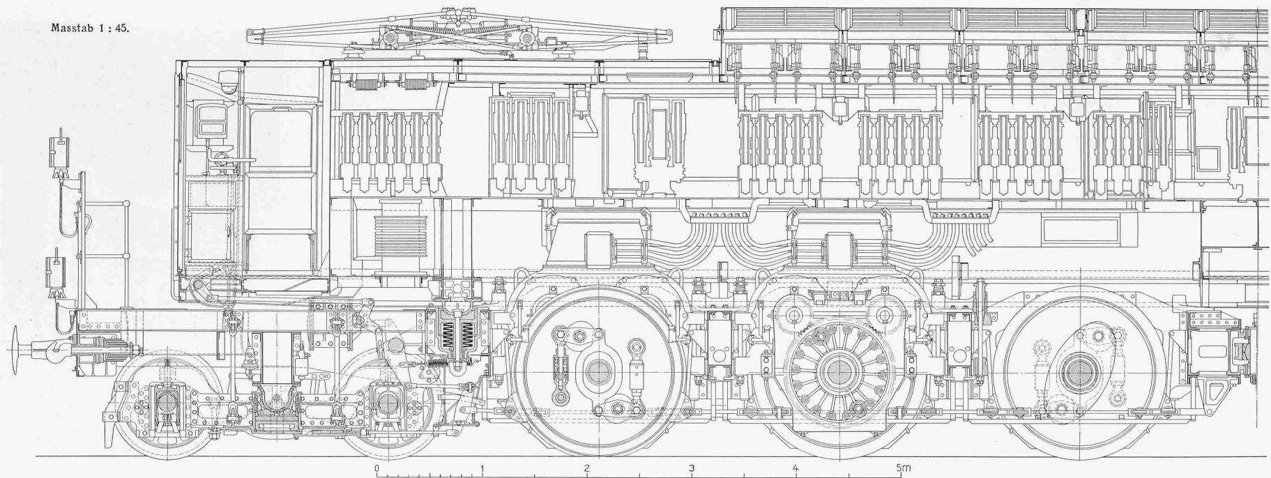
SCHNELLZUGSLOKOMOTIVE VON 5400 PS DER P. L. M.
