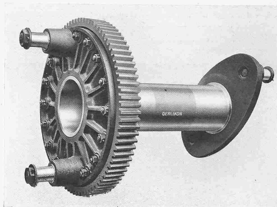
Abb. 3. Hohlwelle mit Kupplungszapfen und Zahnrad.
