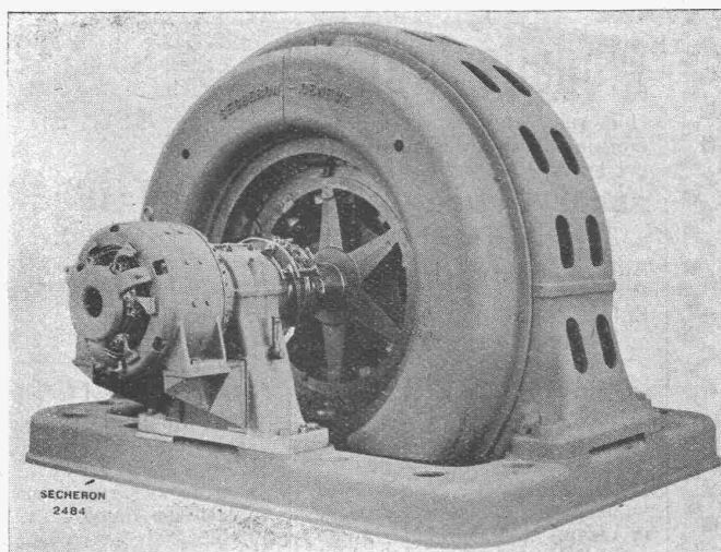
ALTERNATEUR de 3000 kVA environ à 500 t/min pour accouplement à une turbine hydraulique, vitesse d'emballage 1000 t/min.
