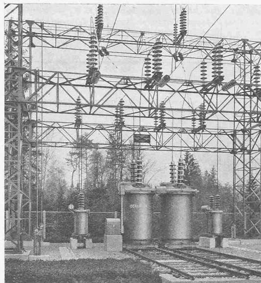
Abb. 8. 132 kV-Oelschaltergruppe mit Spannungswandler 66000/110 V.
