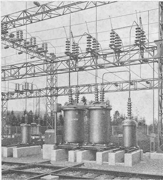
Abb. 9. 66 kV-Oelschaltergruppe mit Stromwandler für 200/5 A.
