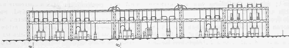
Abb. 7. Längsschnitt und Ansicht der 66 kV-Anlage, aus Osten.
