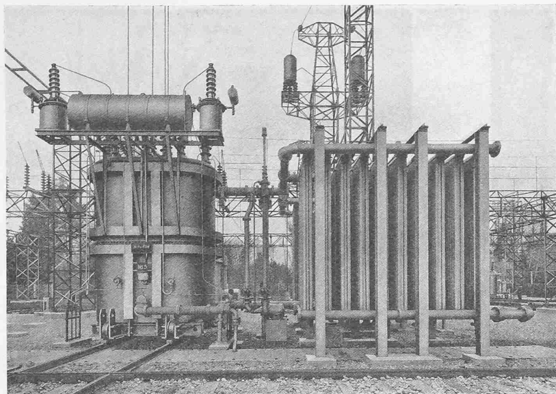
Abb. 10. 9000 kVA-Transformator von der Unterspannungsseite gesehen.
