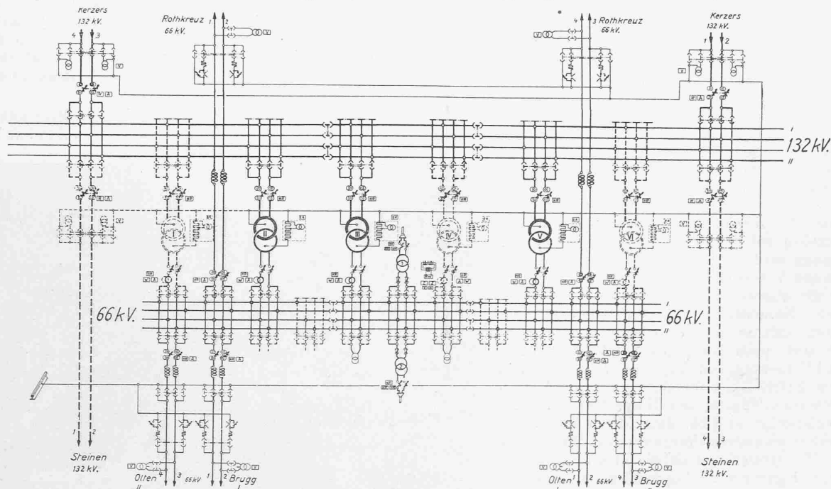
Abb. 3. Schaltungsdiagramm der Freileitungsanlage des Unterwerkes Ruppertswil. — Legende: A Ampèremeter, ER Erdschluss-Relais, H Höchststrom-Relais, NR Nullspannungs-Relais, R Relais-System, RW Registr. Wattmeter, SW Summenstromwandler, V Voltmeter, W Wattmeter, Z Zähler.
